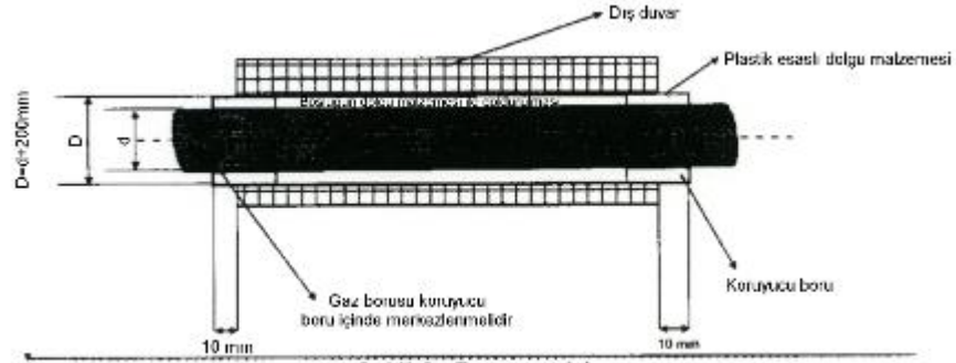
Şekil 9 Duvar Geçiş
