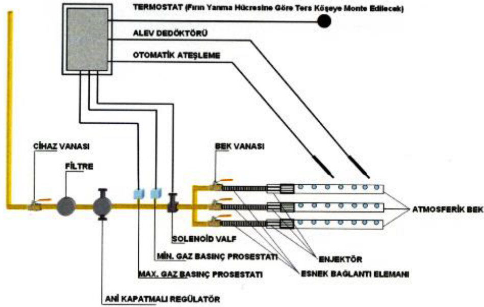
Şekil 27 Fırınlarda brülör emniyet ekipmanları montaj şeması
