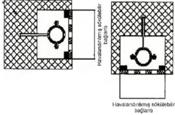
Şekil 10 Duvar/Asma tavan içi kanal ve boru geçiş detayı
